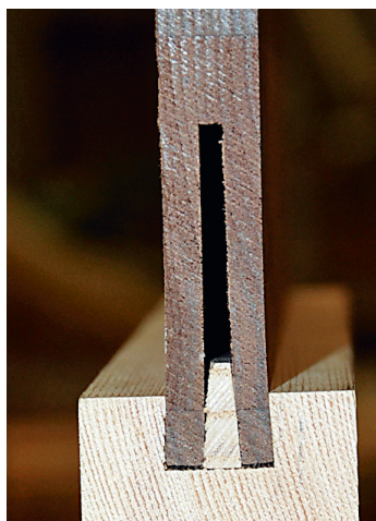
Själva smygen (det mörka träet) har extra djupt spår, så att man kan kapa den efter eget behov.
